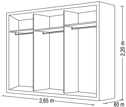
DISTRIBUCIÓN INTERIOR ARMARIO 3 PUERTAS
